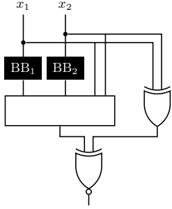
Fig. 3. XOR template
