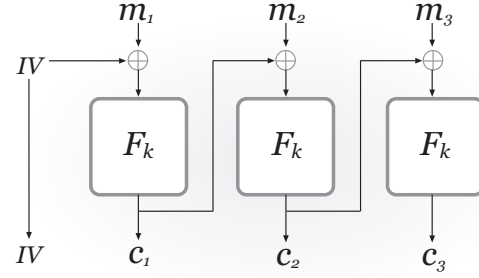
Fig. 1. CBC mode.
